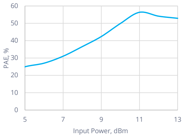
PAE vs. Input Power (F = 2,8 GHz)
